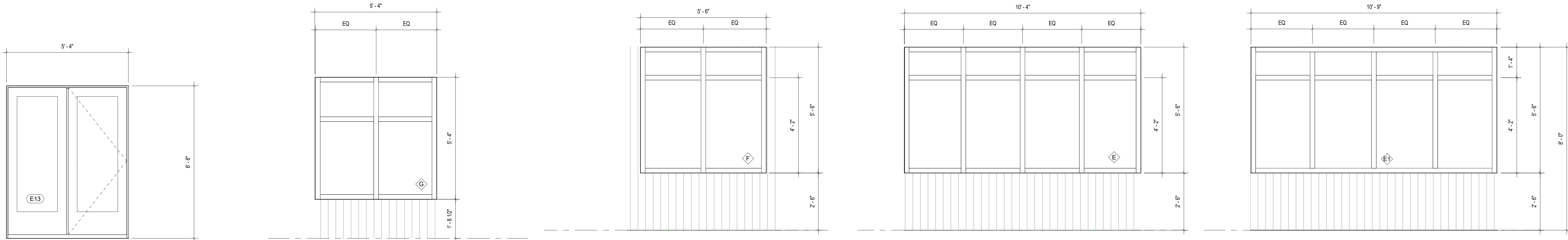
12 PATIO DOOR TYPES E12 AND E13 1/2" = 1'-0"
